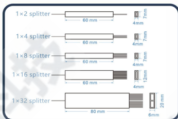
Dimensiones estándar
